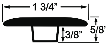
T-Mold
